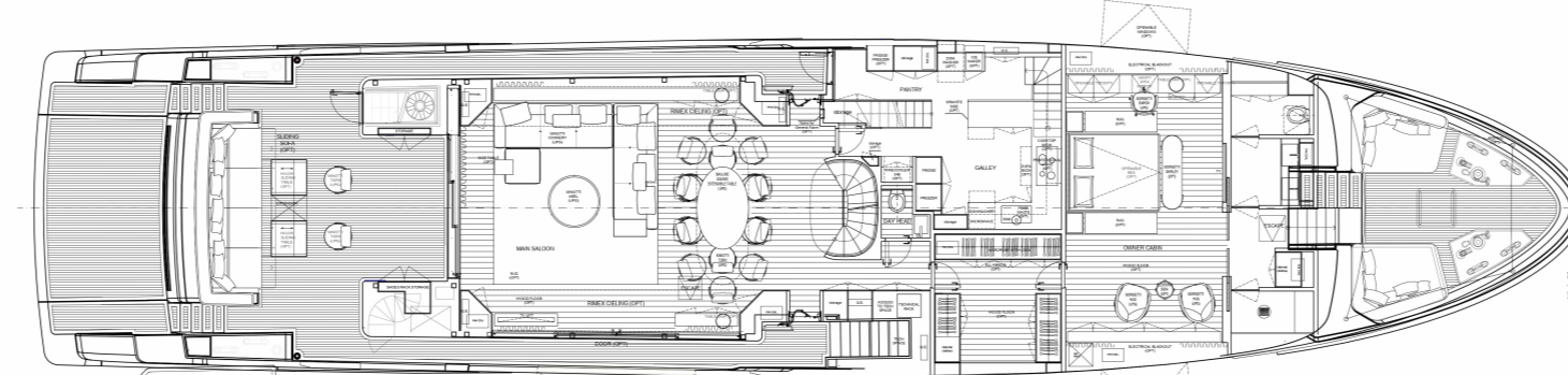
PONTE SUPERIORE UPPER DECK
