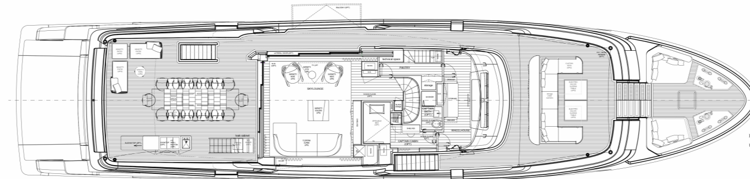
PONTE FLY FLY DECK
